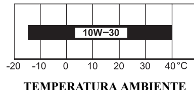
TEMPERATURA AMBIENTE
