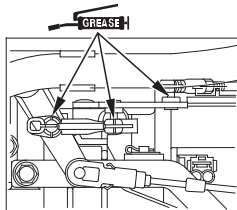
BRAZO DEL ACCELERADOR/ ENLACE/PIVOTE/PLATO
