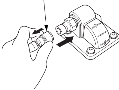
CONECTOR DE LA LÍNEA DE COMBUSTIBLE (AL DEPÓSITO DE COMBUSTIBLE)
