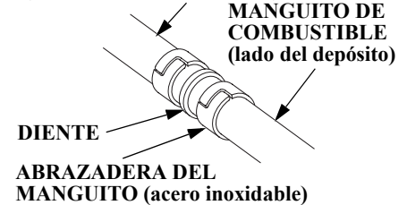
ABRAZADERA DEL MANGUITO (acero inoxidable) (lado del depósito de combustible)
