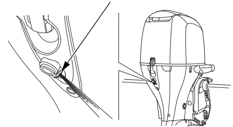
ORIFICIO DE COMPROBACIÓN DEL AGUA DE REFRIGERACIÓN
